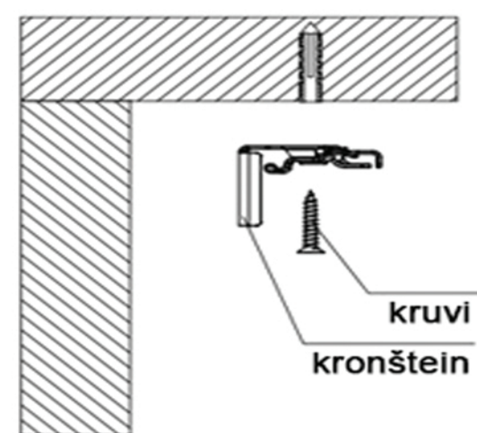
Kinnitamine lakke
